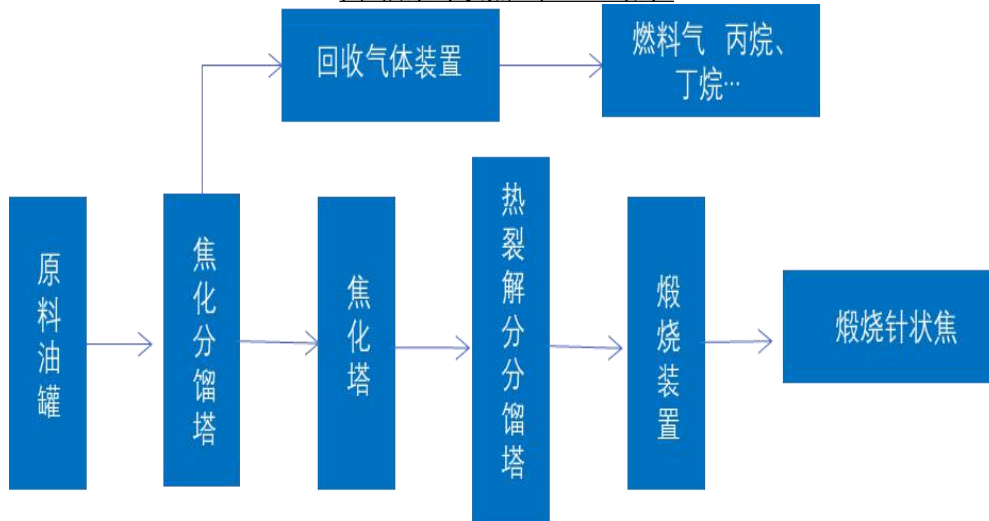
图 油系针状焦生产工艺流程
