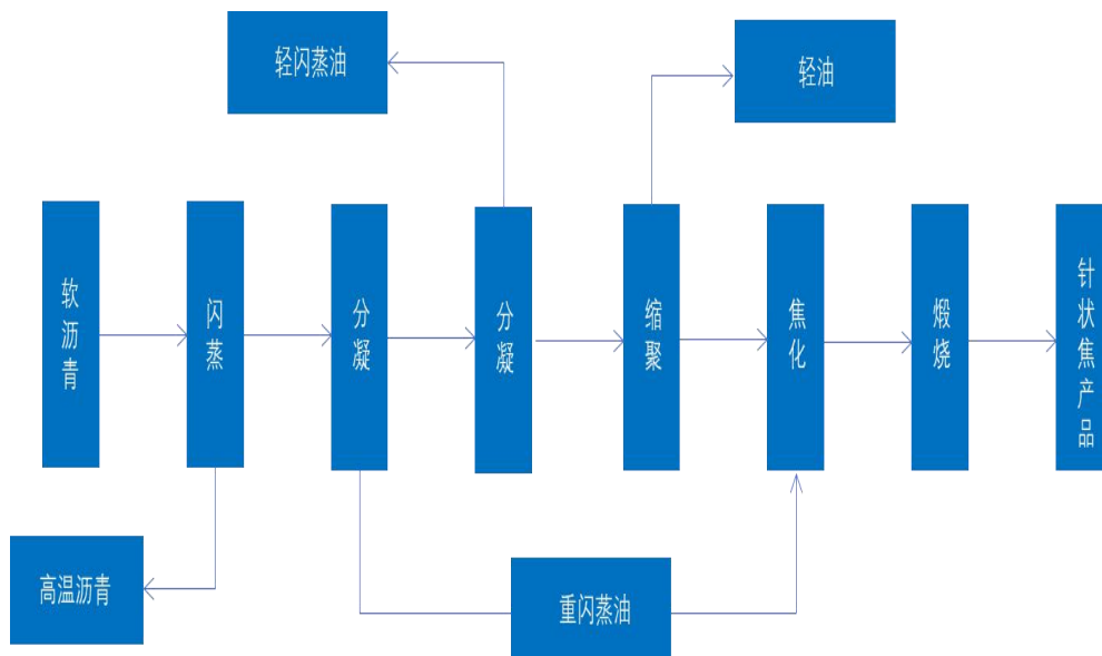
图 煤系针状焦生产工艺流程
