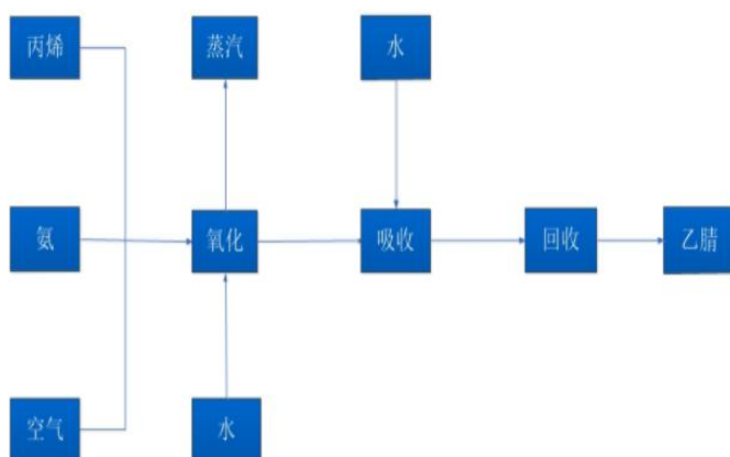
氨氧化副产法乙腈工艺流程图
