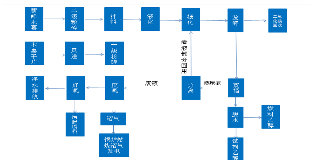
木薯乙醇生产工艺图
