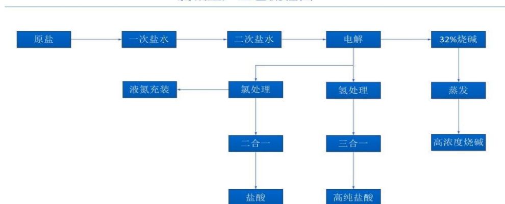
氯碱生产工艺流程图
