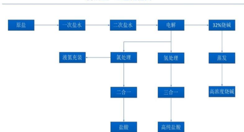
氯碱生产工艺流程图
