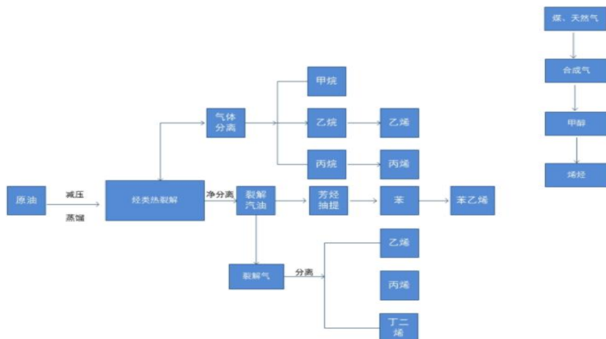
丁二烯工艺流程图
