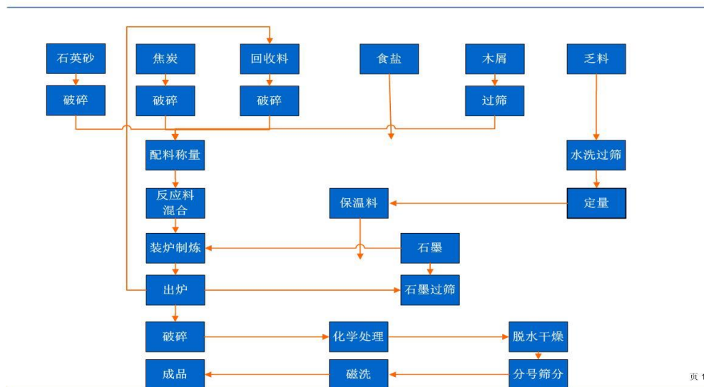
碳化硅生产工艺流程图
