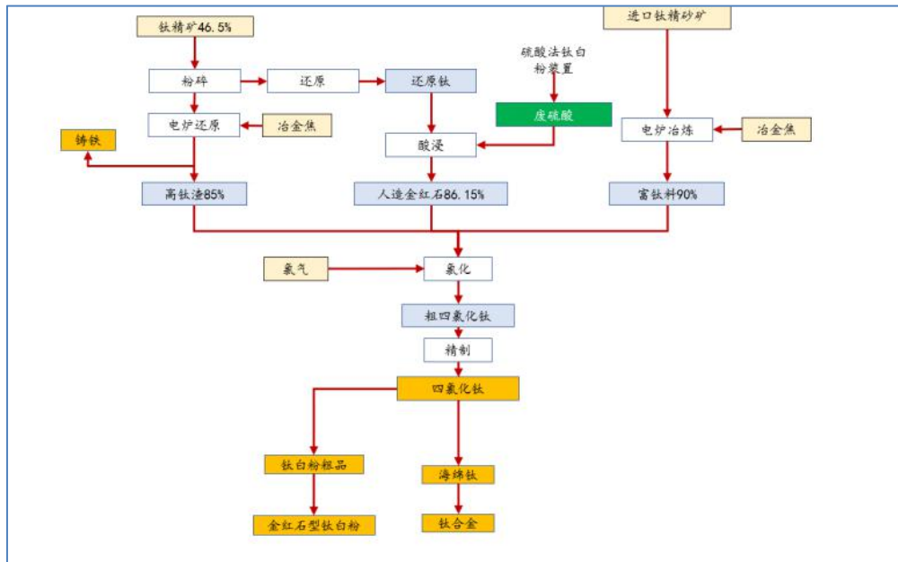
钛产业链工艺流程图
