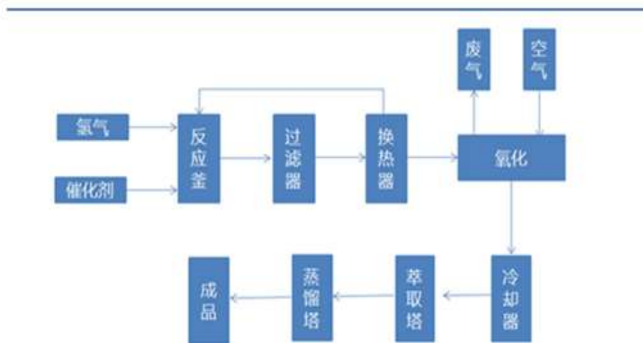
双氧水工艺流程图
