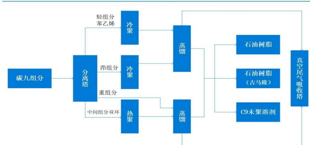
C9石油树脂生产工艺图
