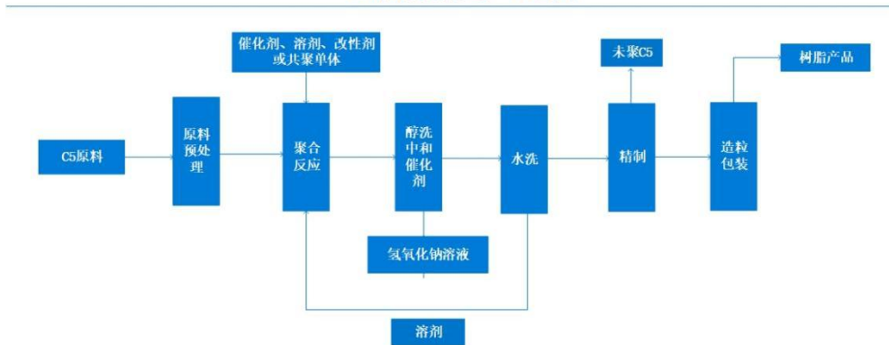
C5石油树脂生产工艺图
