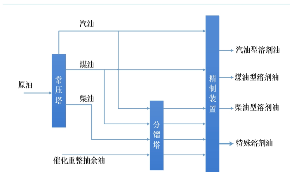
图：溶剂油生产工艺流程图
