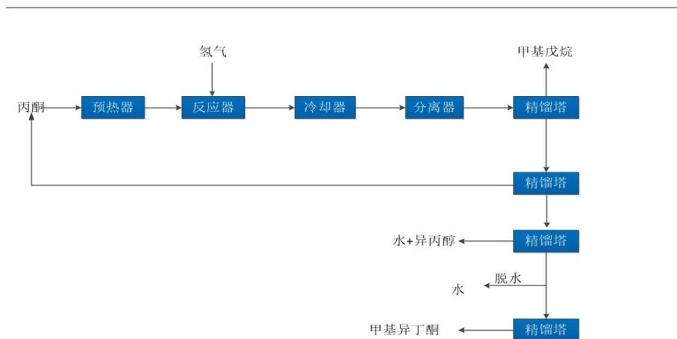
MIBK 丙酮法生产工艺图
