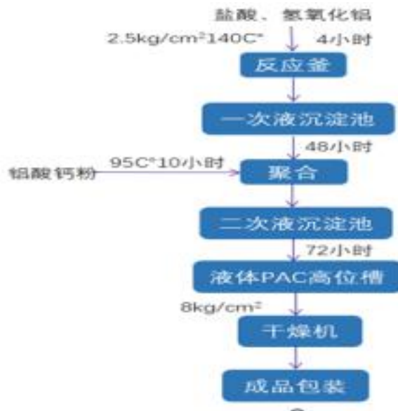
图：聚合氯化铝生产工艺流程图
