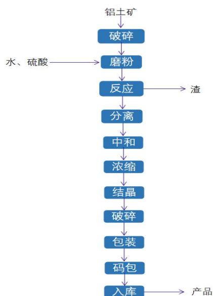
图：硫酸铝生产工艺流程图
