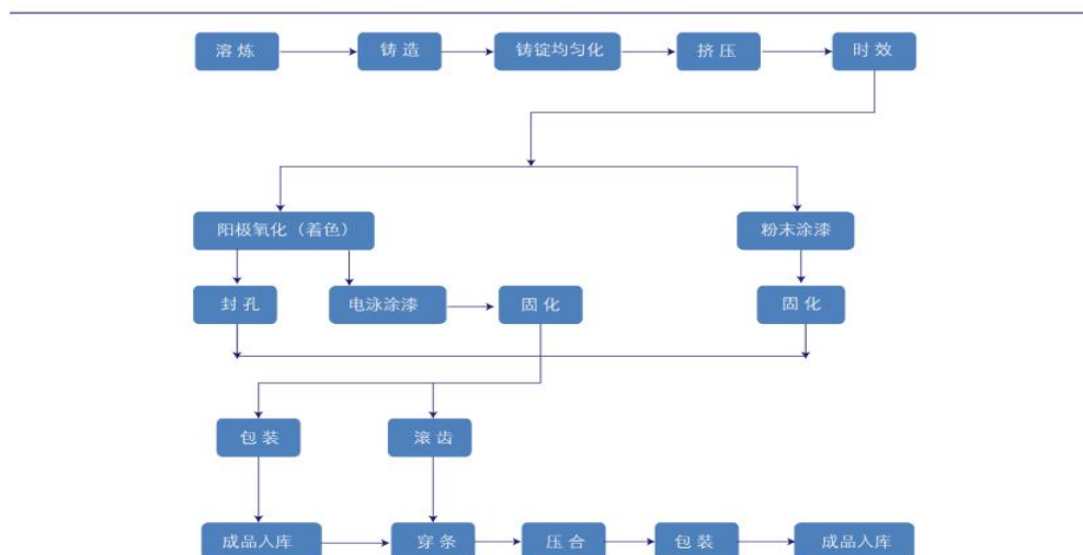
有色—铝加工生产工艺图
