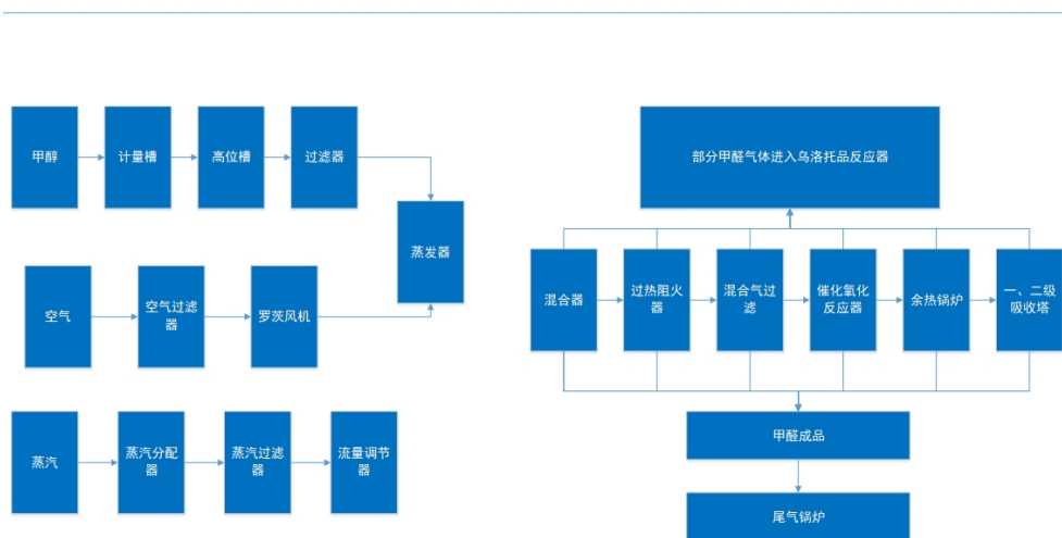
甲醇空气氧化法制甲醛工艺流程图
