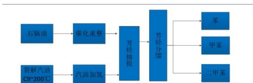
甲苯生产工艺流程图
