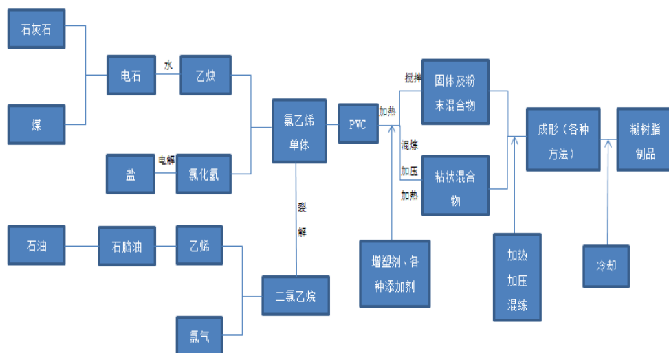
糊树脂生产工艺流程图
