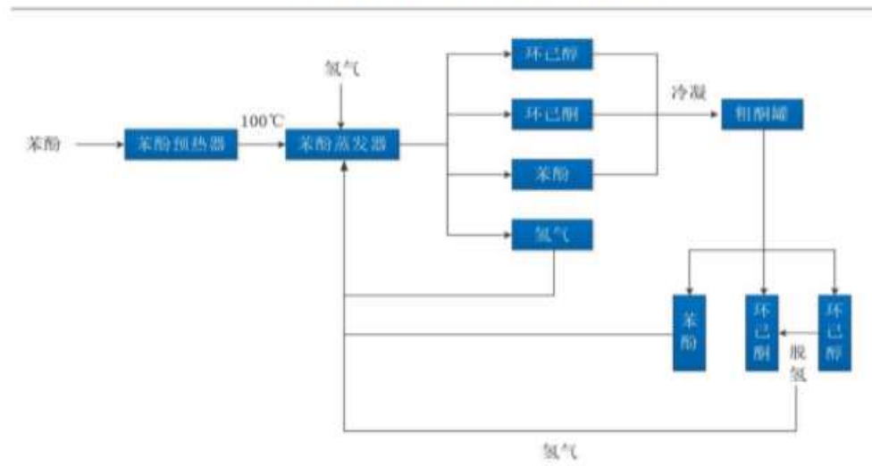
环己酮苯酚加氢法生产工艺图
