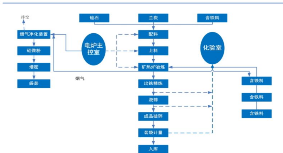
硅铁生产工艺流程图
