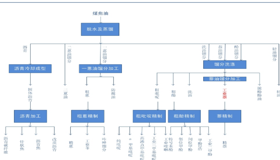
工业萘生产工艺流程图
