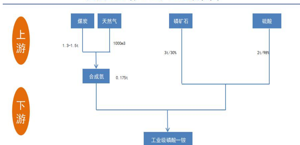
湿法工业级MAP生产工艺流程图
