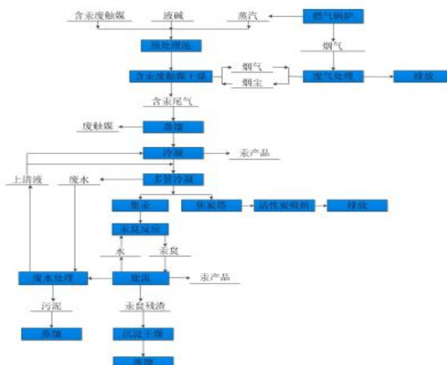
废料回收汞生产工艺流程图
