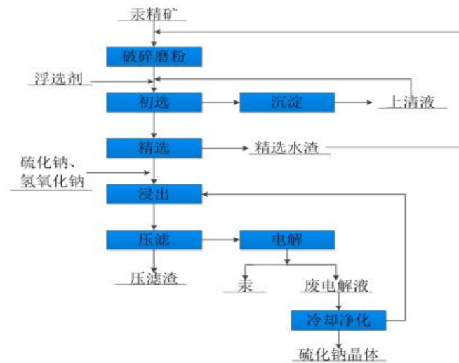
湿法炼汞生产工艺流程图
