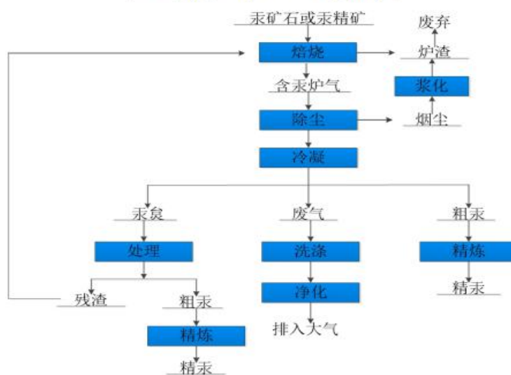
火法炼汞生产工艺流程图
