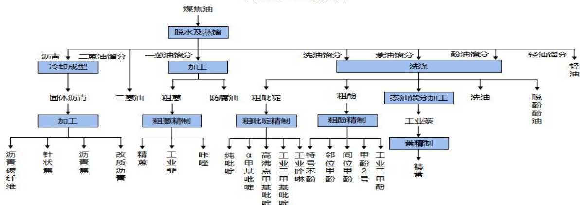
蒽油生产工艺流程图
