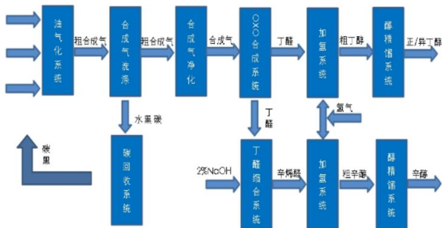
丁辛醇工艺流程图
