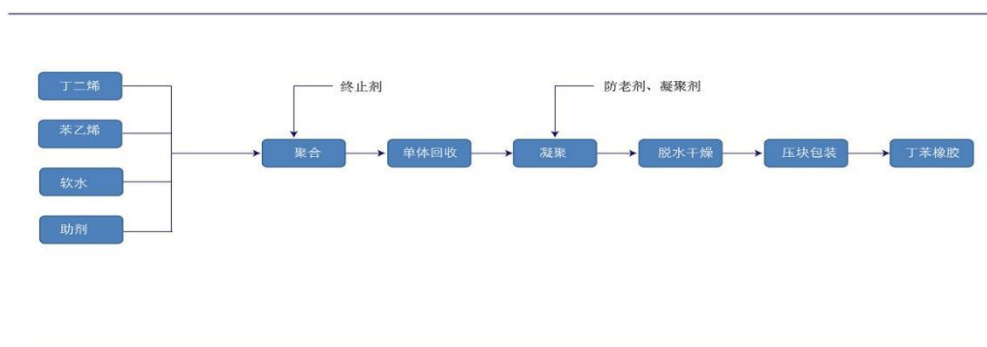
丁苯生产工艺流程图
