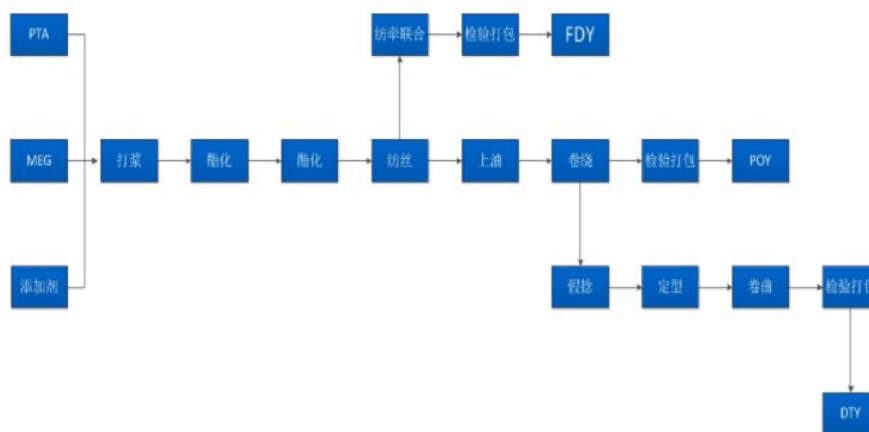
涤纶长丝工艺流程图
