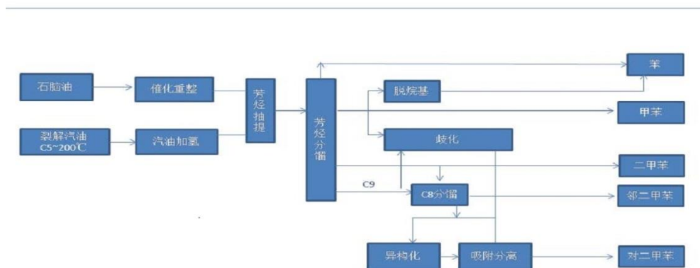
石油制芳烃工艺流程图
