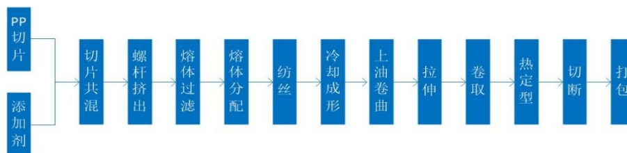
丙纶生产工艺流程图
