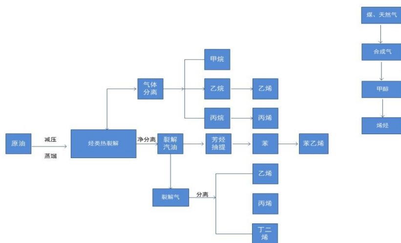
苯乙烯工艺流程图
