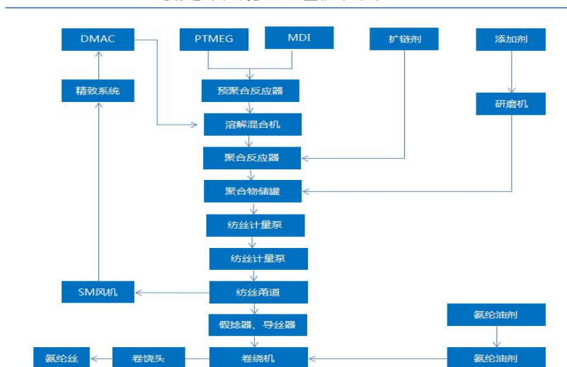
氨纶干法纺丝工艺流程图
